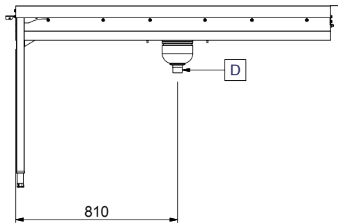
Zij aanzicht
